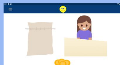
Abbildung 2: Entscheidungsszenario
